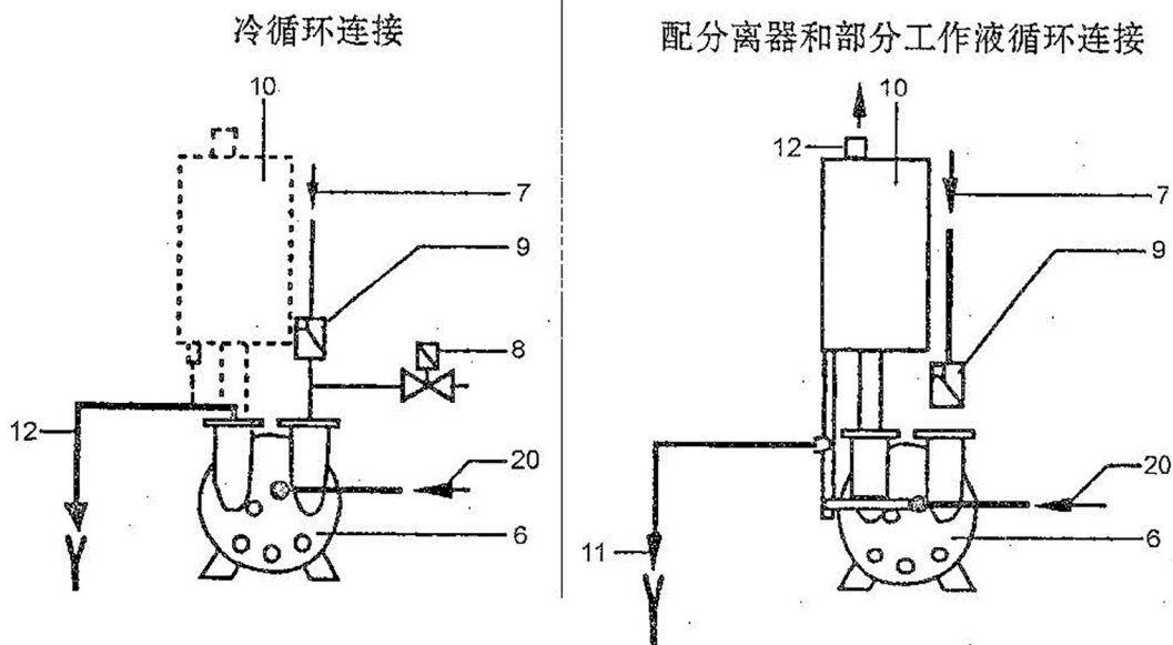
图2 工作液连接 (推荐)
