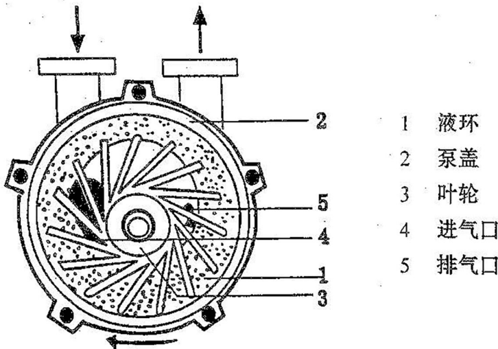
图1 切过泵体的剖视图（向泵盖端看）
