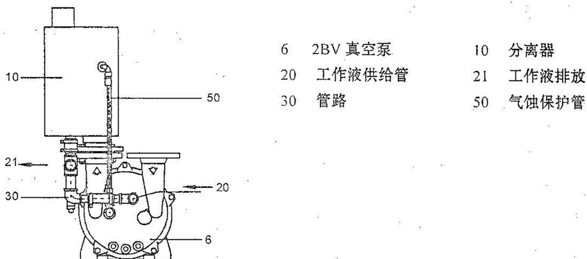
图4 真空泵带分离器和气蚀保护
